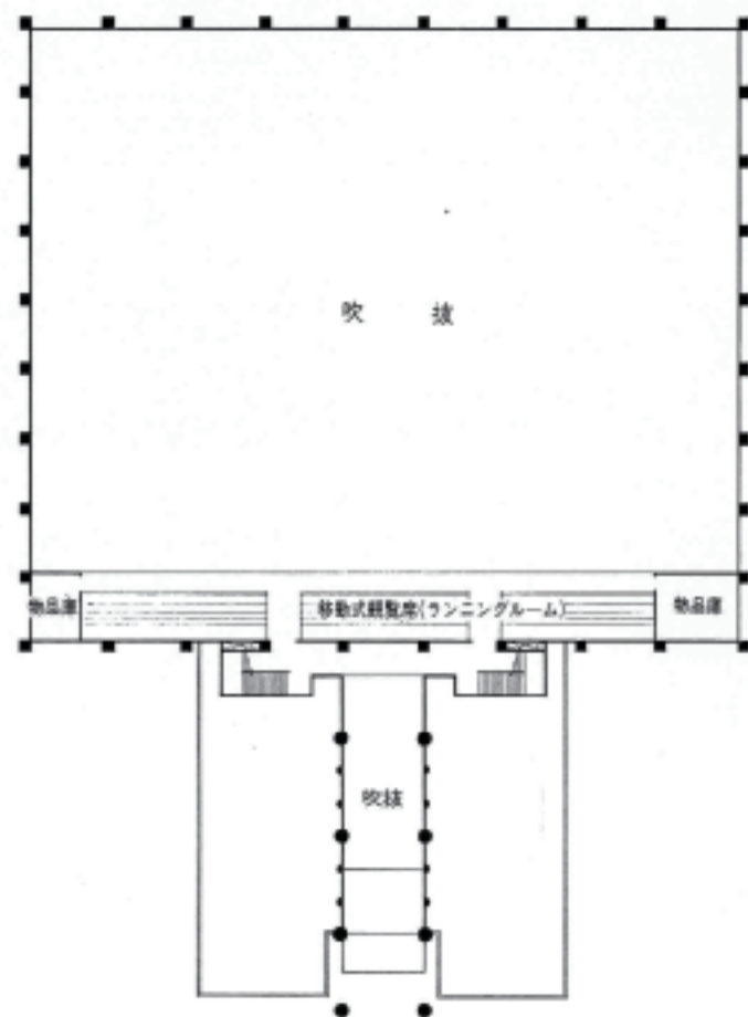
2階平面図
